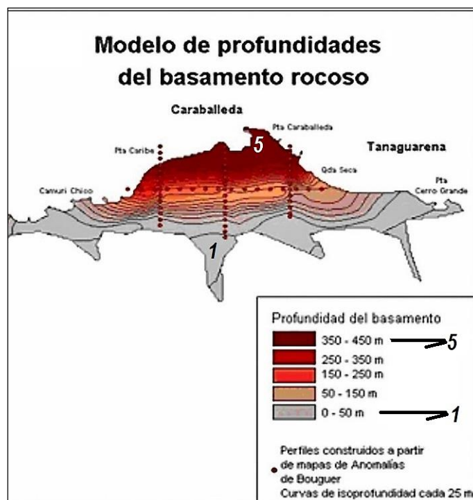
Figura 7. Modelo de profundidades del basamento rocoso del abanico aluvial de Caraballeda (Estado La Guaira, Venezuela), generado a partir de curvas de isoprofundidad (equidistancia 25 m) e inversión de anomalías gravimétricas de Bouguer. La escala de colores indica la profundidad del basamento desde facies someras (0-50m) hasta la depocentral máxima (350-450 m).
